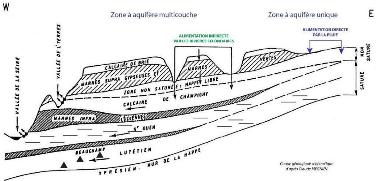
Figure 3 : Coupe géologique schématique de la Brie
