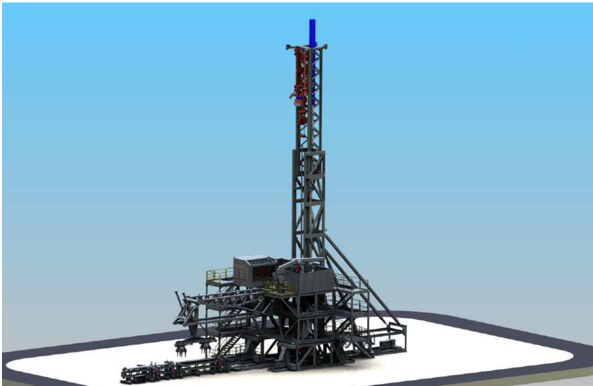
Figure 11: Schéma d'un rig électrique en co-construction, (Source : Herrenknecht Vertical GmbH)
