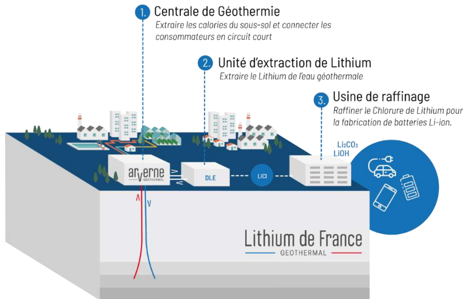
Figure 9: Schéma d'implantation d'une centrale géothermique et l'unité d'extraction de Lithium envisagés par Lithium De France (source : Lithium de France).
